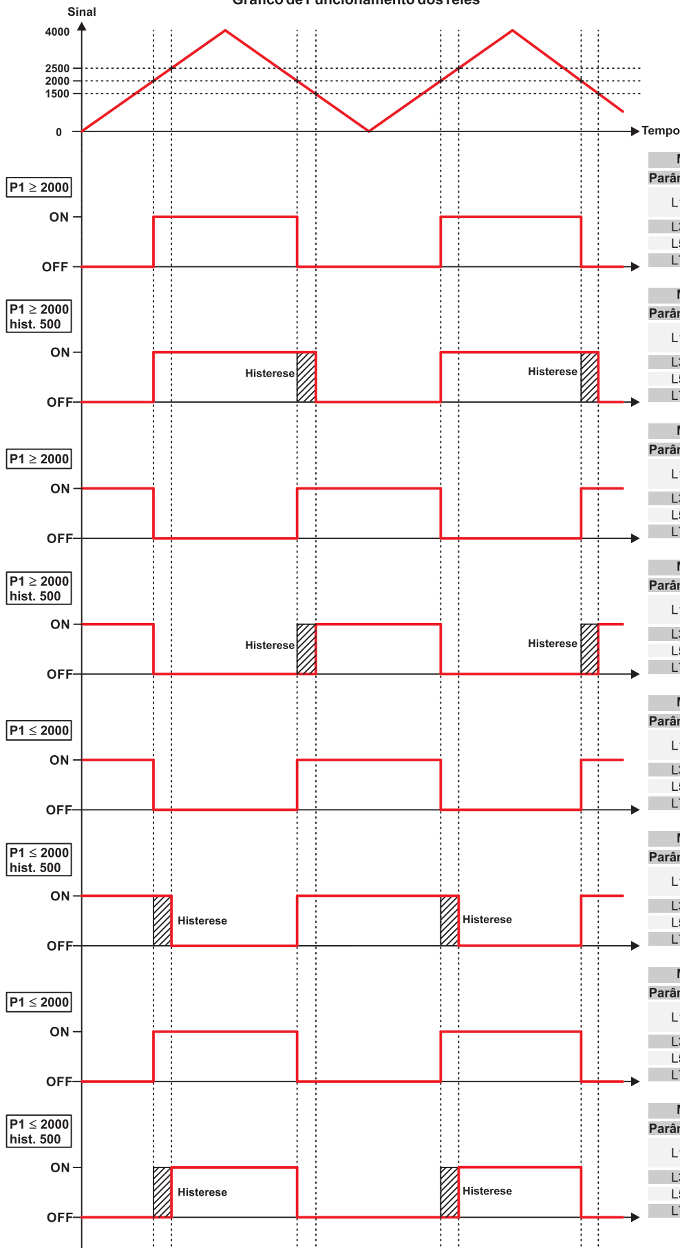
Gráfico de Funcionamento dos relés
